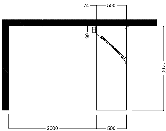
Zij aanzicht
